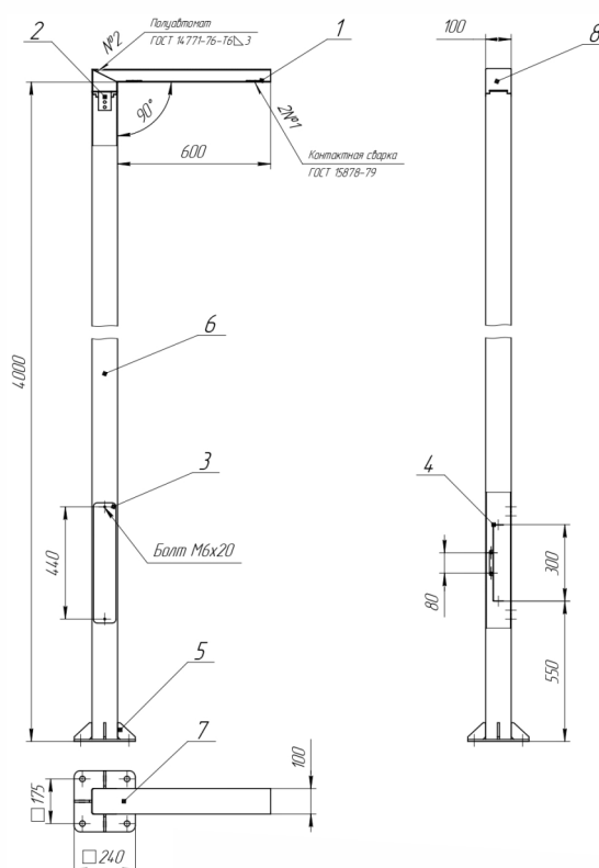
Опора П-100х50-3, О-5000-Т
