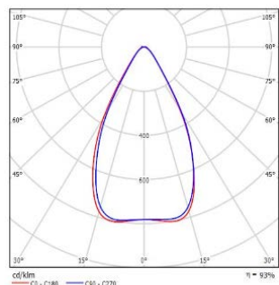
Тип КСС: «Г» - 60°
