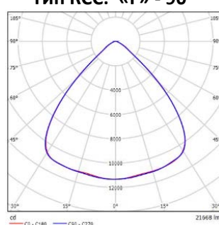
Тип КСС: «Г» - 90°
