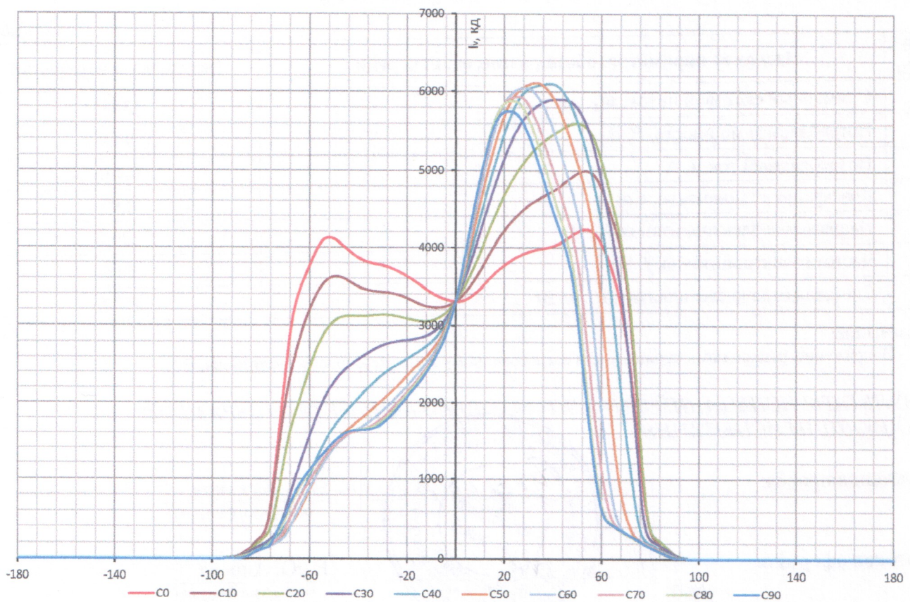
Рисунок 2. Декартовы координаты
